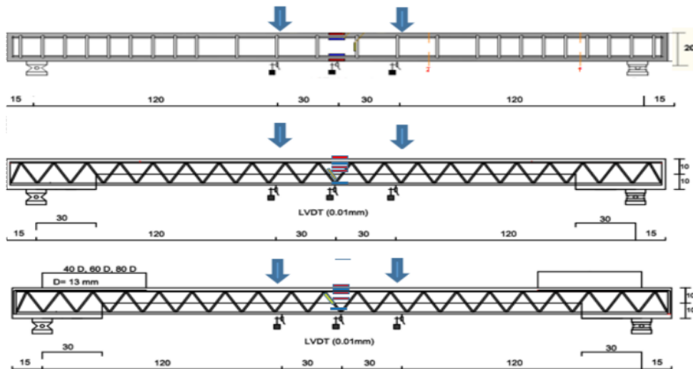
Gambar 5. Set Up Pengujian
