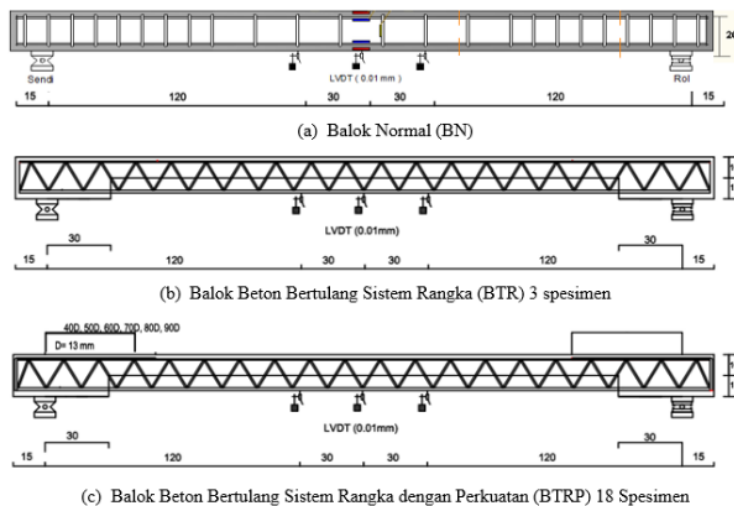
Gambar 3. Spesimen Balok
