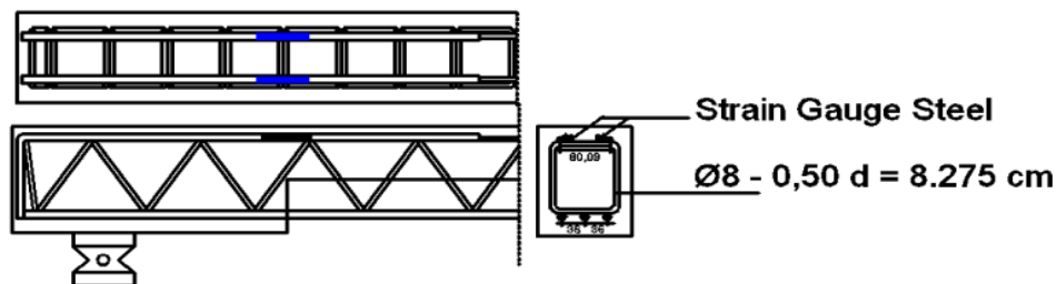
Gambar 4. Tulangan Tarik Perkuatan
