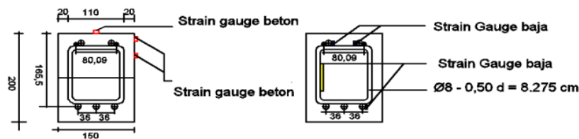
Gambar 6. Letak Instrumental
